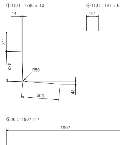
鉄筋加工図
