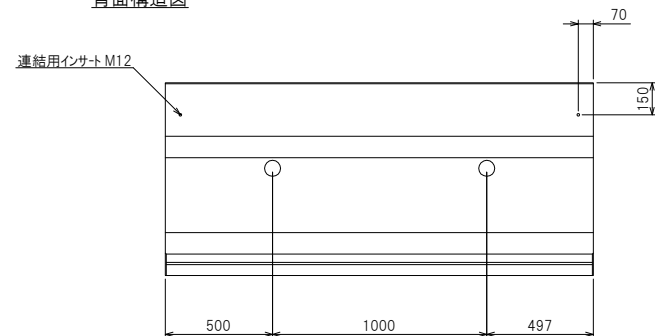
背面構造図
