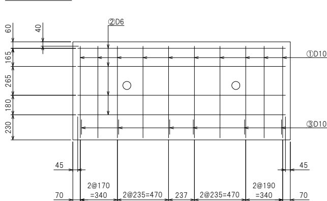
たて壁配筋図
