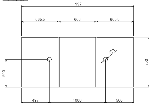
正面構造図
