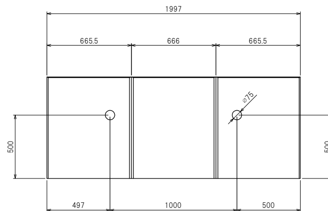
正面構造図
