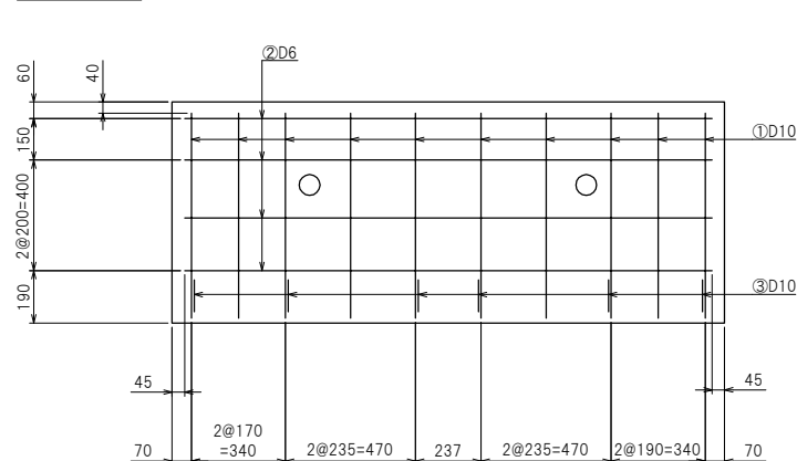
たて壁配筋図
