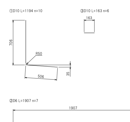
鉄筋加工図
