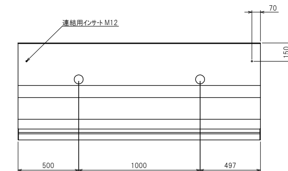
背面構造図
