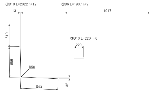
鉄筋加工図
