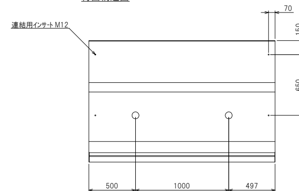
背面構造図
