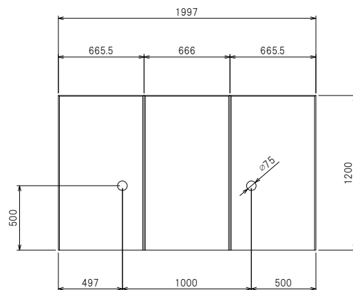
正面配筋図
