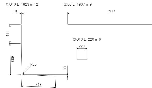
鉄筋加工図
