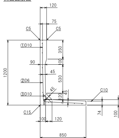
側面配筋図
