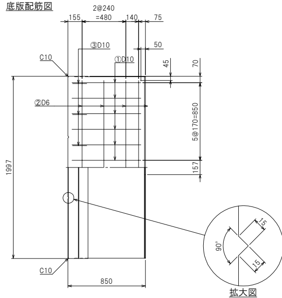
底板配筋図
