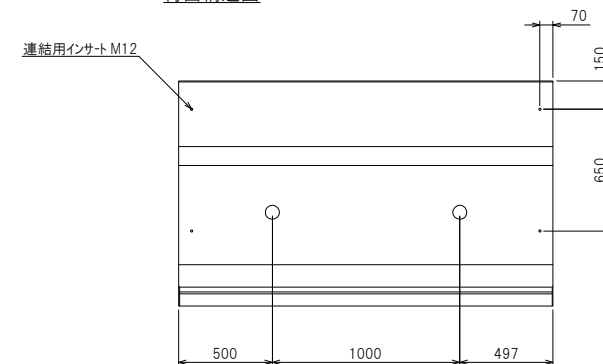
背面構造図
