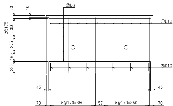
たて壁配筋図
