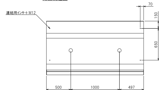
背面構造図
