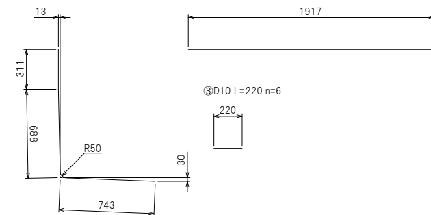
鉄筋加工図
