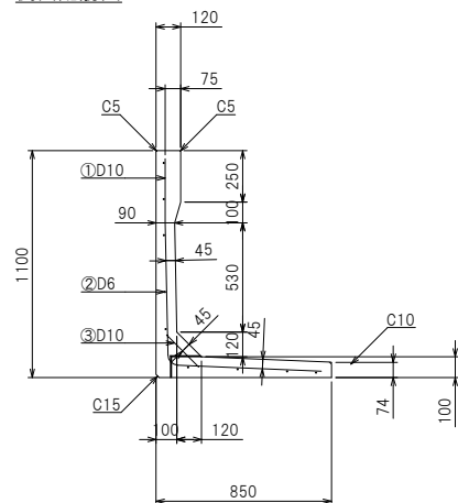
側面配筋図
