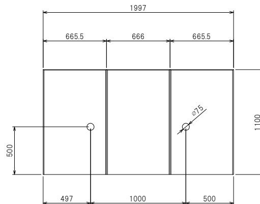
正面配筋図
