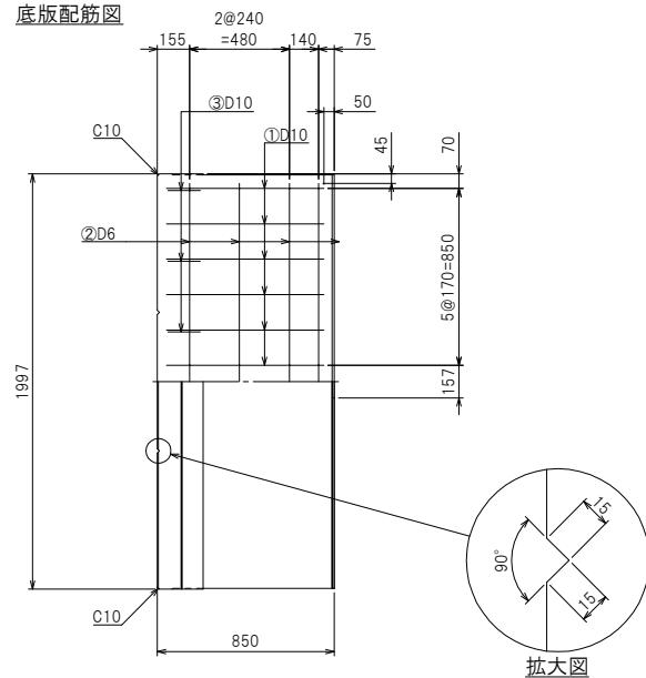
底板配筋図
